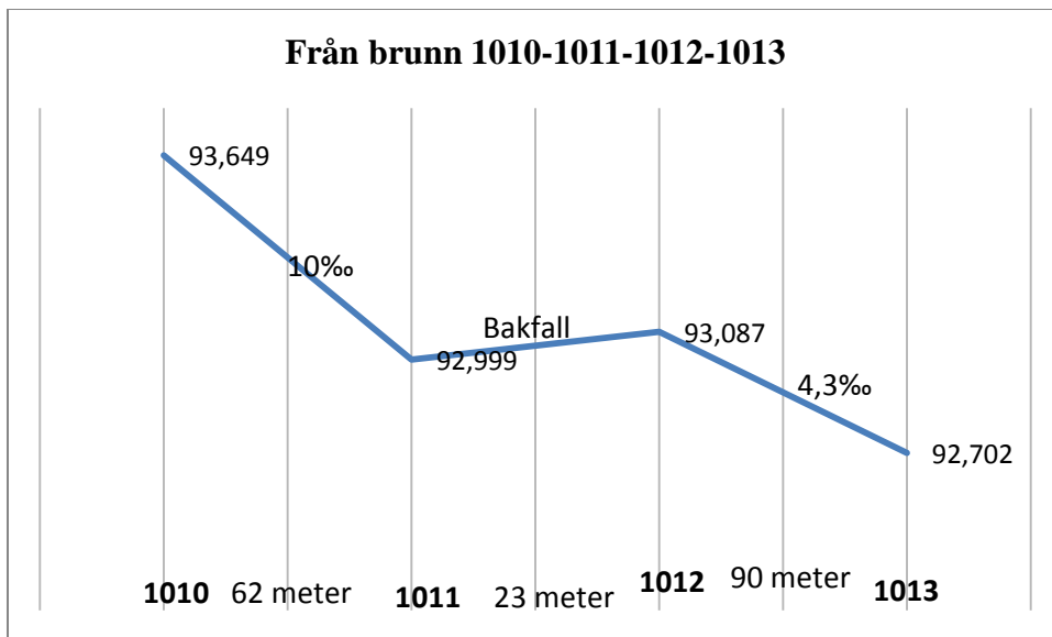
Figur 4. Befintlig vattengång och ledningslutning
