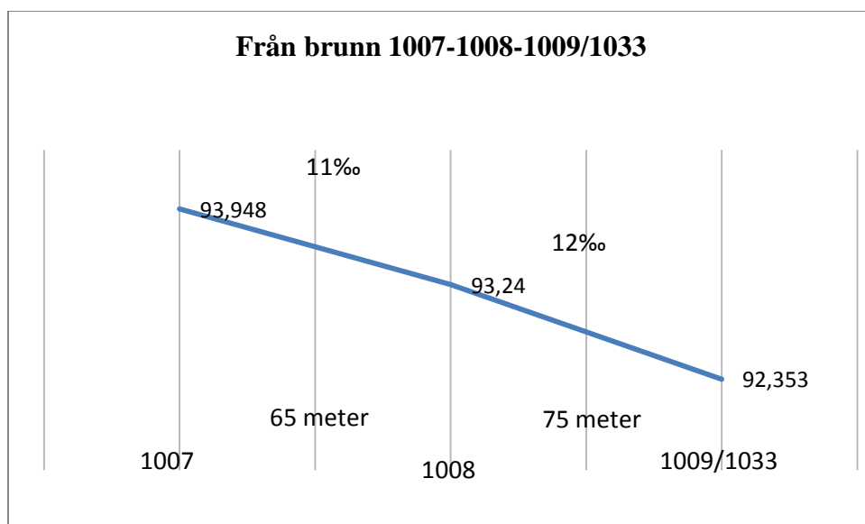
Figur 15. Eventuell vattengång och ledningslutning
